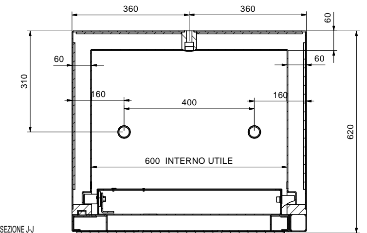
SEZIONE J-J
