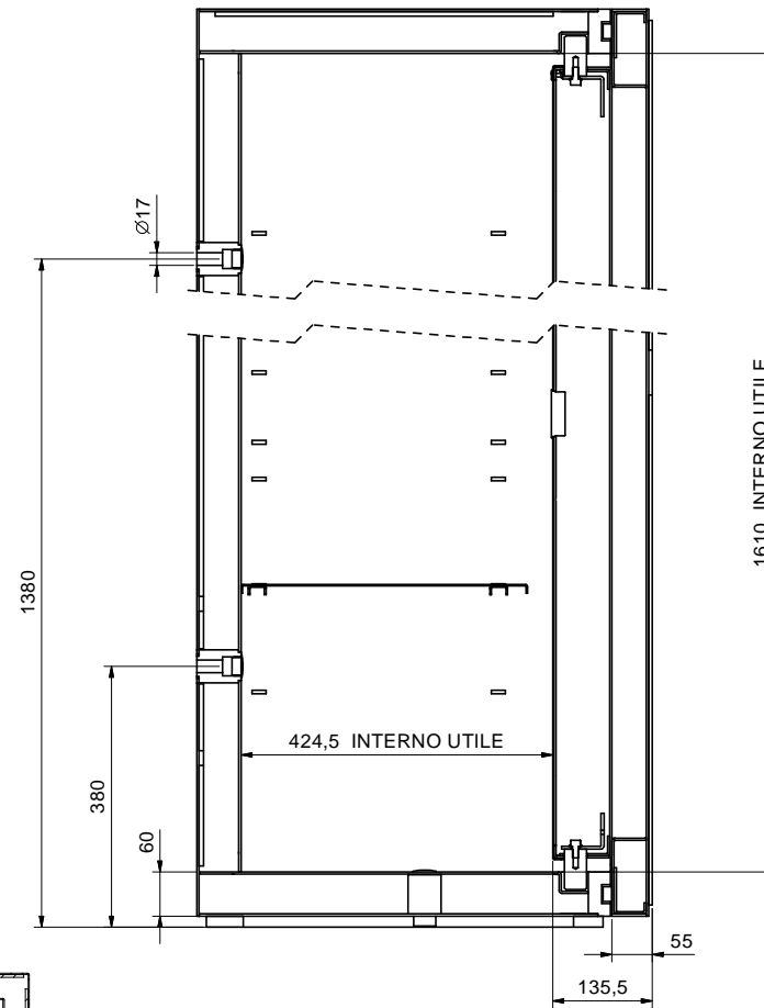
SEZIONE H-H
