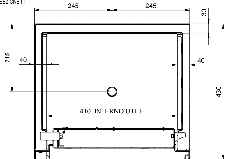
SEZIONE I-I
