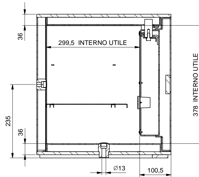
SEZIONE H-H
